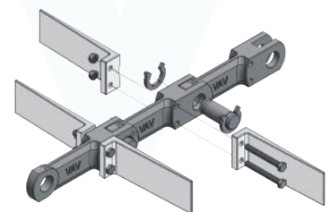
Met eenvoudig te monteren kunststof meenemers
