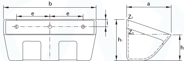
Kunststof elevatorbeker type M (afmetingen in mm)
