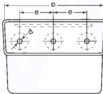
Columbus Elevatorbecher aus Kunststoff (Abmessungen in Mm)
