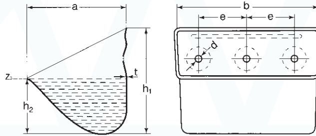
Columbus Elevatorbecher aus Stahl (Abmessungen in mm)
