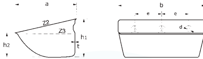
Super Starco Elevatorbecher aus Stahl / Edelstahl (Abmessungen in mm)
